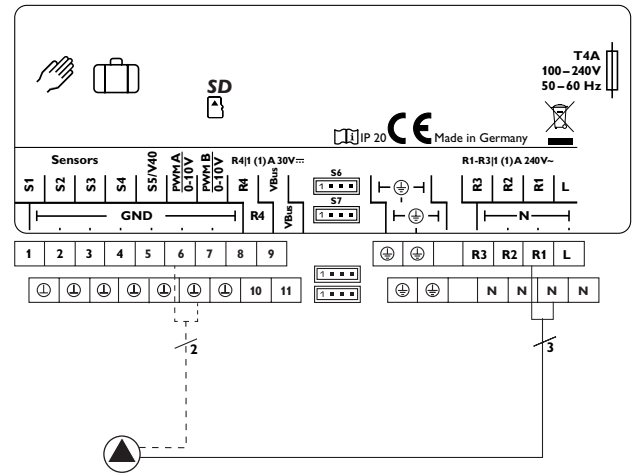
Beispiel für den elektrischen Anschluss einer Hocheffizienzpumpe
